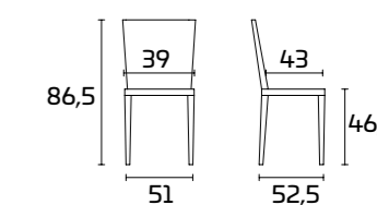
Kuadra 1158 на ползьях
