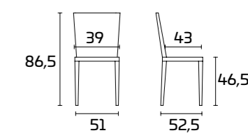
Kuadra 1158 de patín
